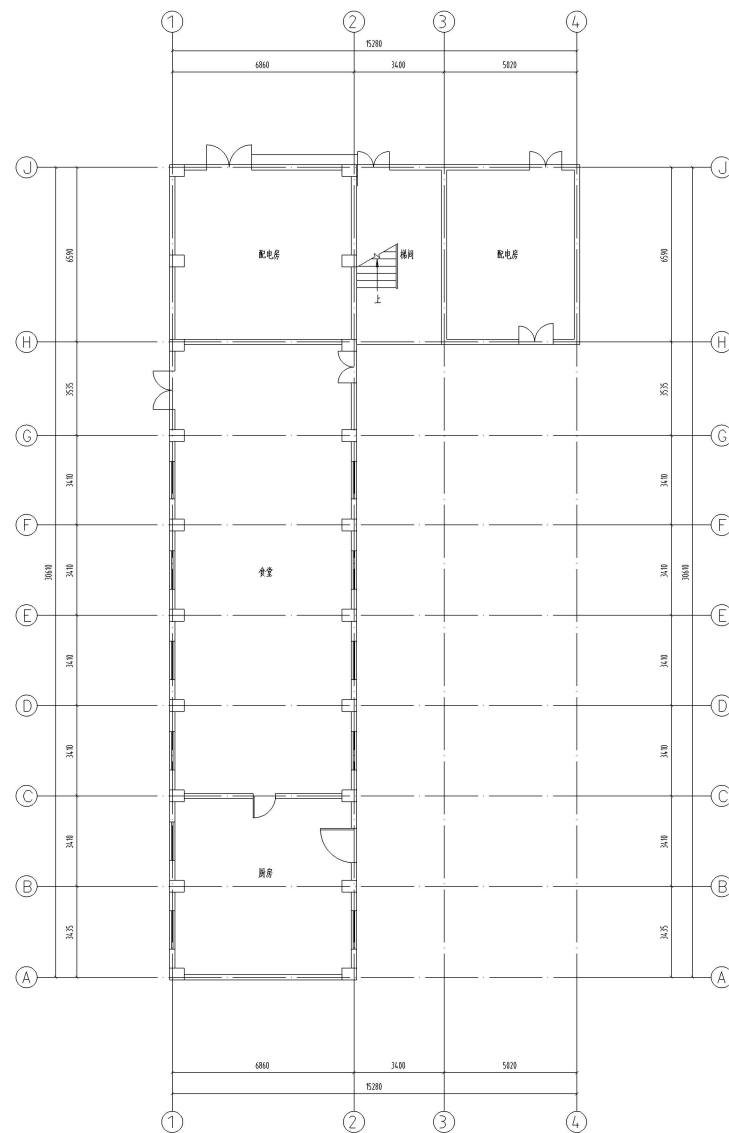
115 栋一层平面图 1:200
